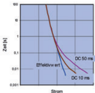
Bild 5.6.4 – Gleichstromkennlinien
