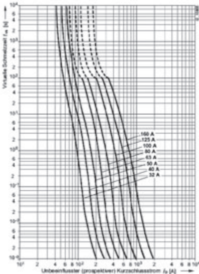
Bild 5.5.4 – Zeit/Strom-Kennlinien von SITOR gR- und aR-Sicherungseinsätzen
