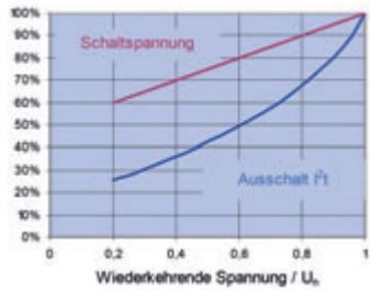
Bild 5.5.3 – Korrektur der Schaltspannungs- und Ausschaltintegrale
