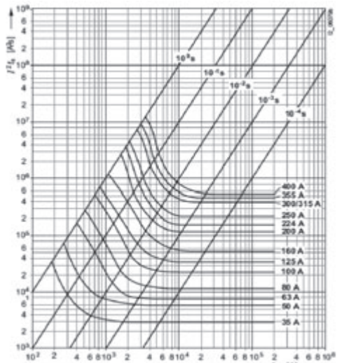
Bild 4.3.3 – I^2t -Kennlinien
