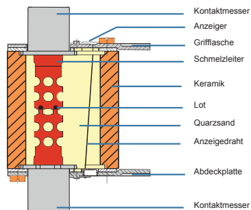
Bild 3.2.2 - NH-Sicherungseinsatz
