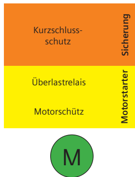
Bild 5.4.1 – Motorstromkreisschema
