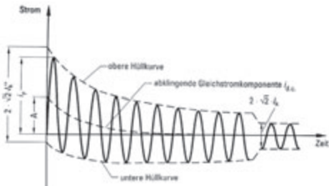
Bild 4.3.5 Kurzschlussstromverlauf im Drehstromnetz
