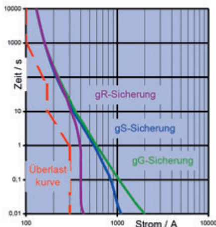
Bild 5.5.2 – Kennlinien gG, gS und aR mit Überlastkurve
