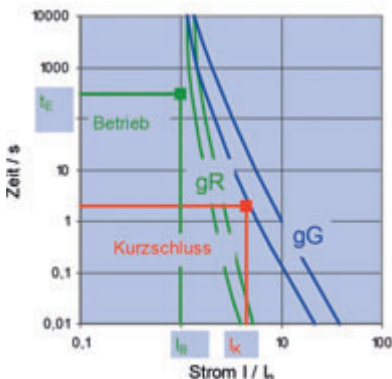
Bild 5.7.2 – Auswahl einer Batteriesicherung für USV-Anlagen
