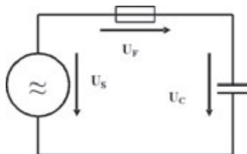
Bild 5.8.3 – Schaltbild kapazitiver Stromkreis
