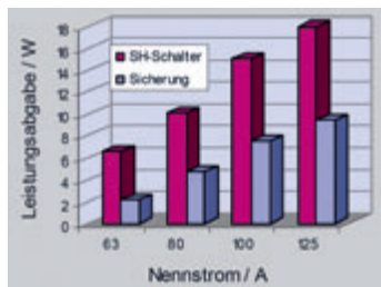
Bild 4.5.2 – Leistungsabgabewerte
