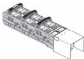
Bild 5.9.2 – Zwillingschaltleiste
