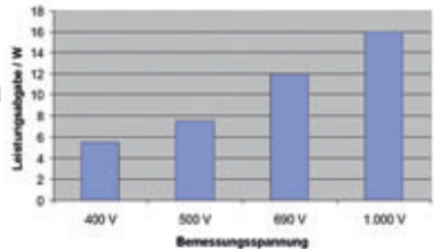
Bild 4.5.4 – Leistungsabgabe von 100 A gG-Sicherungseinsätzen
