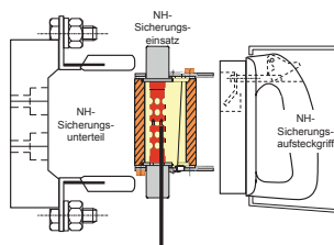
Bild 3.2.1 - NH-Sicherung
