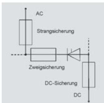
Bild 5.5.1 – Halbleiterschutz, Stromkreisschema
