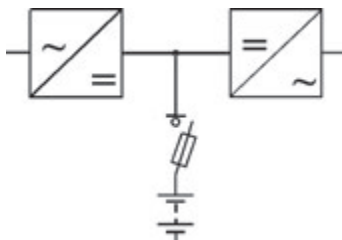
Bild 5.7.1 – Schaltschema einer USV-Anlage
