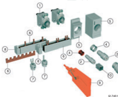
Bild 3.1.9 – NEOZED-Systemkomponenten
