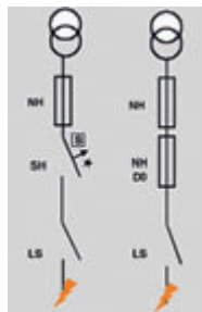
Bild 4.4.4 – Selektivschutz im Hausanschluss
