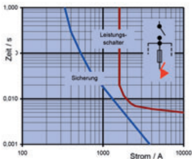
Bild 4.4.2 – Leistungsschalter vor Sicherung
