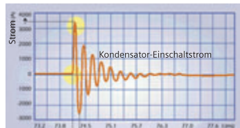
Bild 5.8.2 – Kondensator-Einschaltstrom
