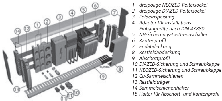
Bild 3.3.5 – Sammelschienensystem SR60
