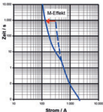
Bild 4.1.6 – Wirkung des Lots auf die Zeit/Strom-Kennlinie
