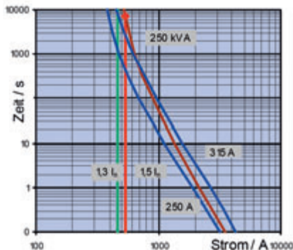
Bild 5.3.1 – Optimaler Transformatorschutz mit gTr-Sicherungen
