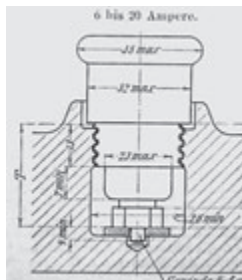
Bild 2.3 – DIAZED-Maßnorm
