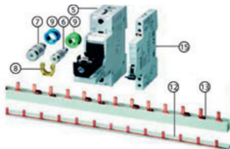
Bild 3.6.5 – MINIZED-Lasttrennschaltersystem D02
