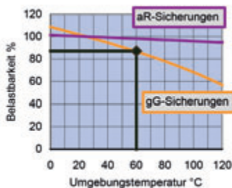
Bild 5.9.1 – Belastbarkeit von Schmelzsicherungen
