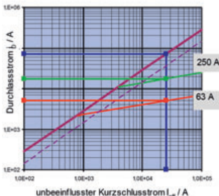
Bild 4.3.4 – Durchlassstrom-Kennlinien
