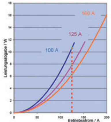
Bild 4.5.5 – Leistungsabgabe von gG-Sicherungen unterschiedlicher Nennströme
