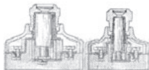
DIAZED mit Passschraube
