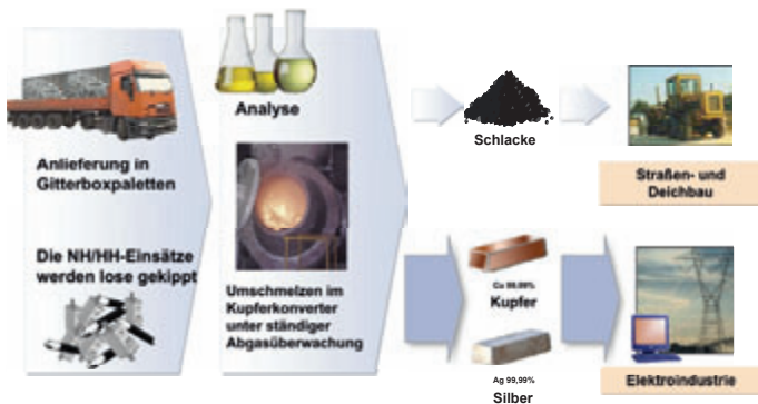
Bild 3.8.5 Recyclingverfahren für NH- und HH-Sicherungen
