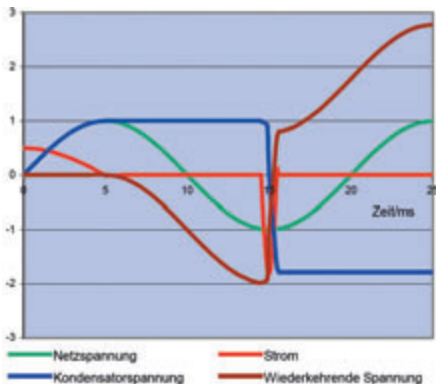
Bild 5.8.4 – Kondensatorabschaltdiagramm
