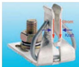
Bild 3.2.7 – Lyrakontakt eines NH-Unterteils
