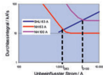
Bild 4.4.5 – Selektivitätsgrenzen
