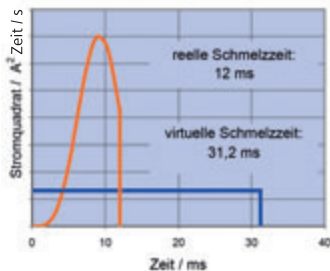
Bild 4.3.2 – Reelle und virtuelle Zeiten
