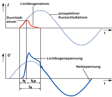
Bild 4.1.3 – Kurzschlussstrombegrenzung
