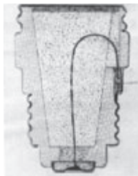
Bild 2.1 – Schmelzstößel mit Edisongewinde (um 1900)
