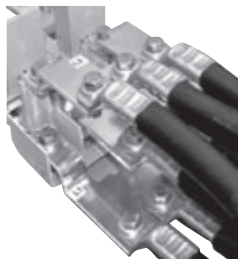
Bild 5.9.3 – Kabelanschlussbereich
