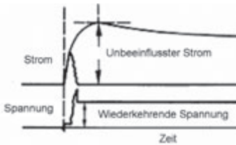
Bild 5.6.2 – DC-Kurzschlussabschaltung
