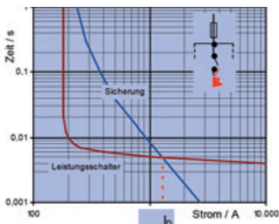
Bild 4.4.3 – Sicherung über Leistungsschalter
