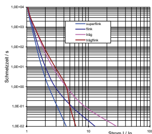
Bild 3.1.4 – DIAZED®-Charakteristiken
