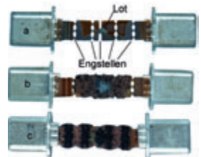
Bild 4.1.4 – NH-Schmelzleiter a) neu, b) nach Überlastabschaltung, c) nach Kurzschlussabschaltung
