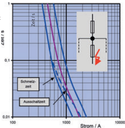
Bild 4.4.1 – Selektiver Schutz im Strahlennetz
