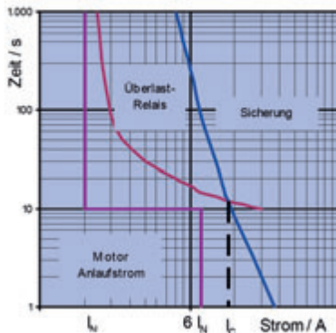
Bild 5.4.2 – Auswahl von Motorschutzsicherungen
