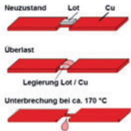
Bild 4.1.5 – Lotreaktion bei Überlastabschaltung
