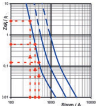
Bild 4.3.1 – Zeit/Strom-Kennlinien
