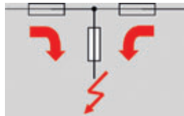
Bild 4.4.6 – Knoten im Maschennetz
