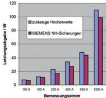
Bild 4.5.4 – Leistungsabgabe von NH-Sicherungseinsätzen
